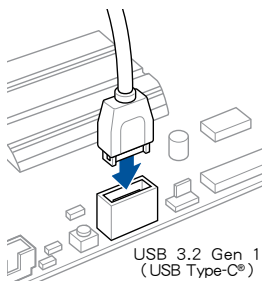
安装 USB 3.2 Gen 1 连接插座 (USB Type-C®)
